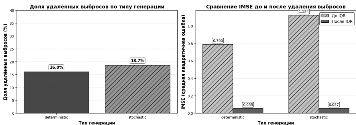
Рис. 45. Влияние очистки от выбросов на смешанных данных для энтропийного метода.
